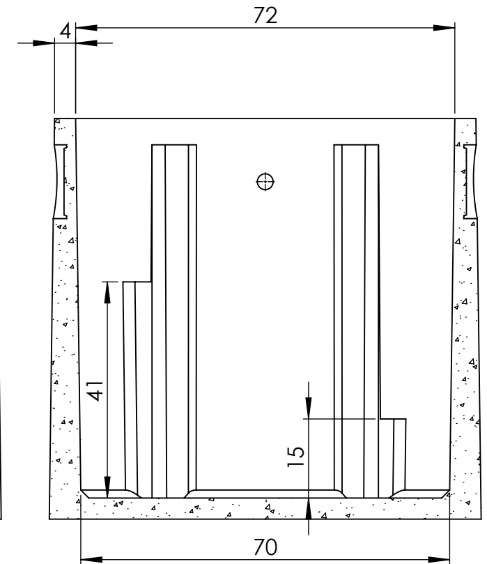
COUPE F-F
