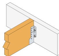
Valeurs caractéristiques - Bois sur béton ou acier
