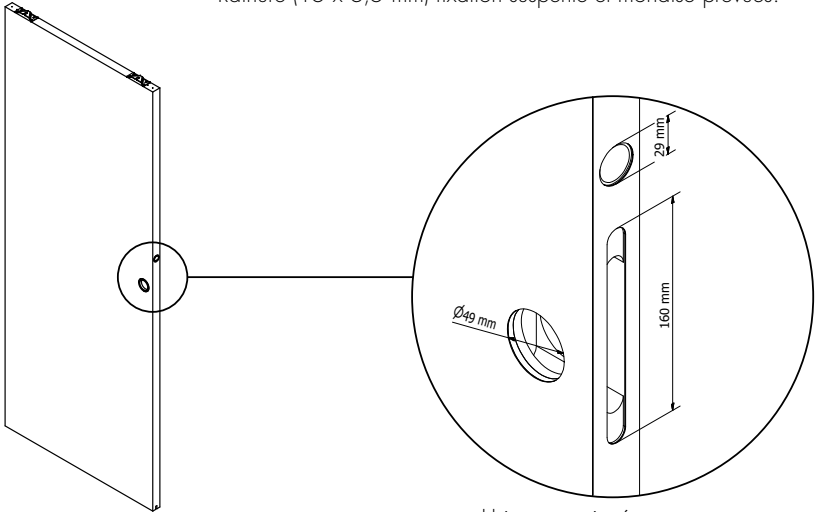
Usinages poignées ou serrure
