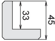
cornière 45
